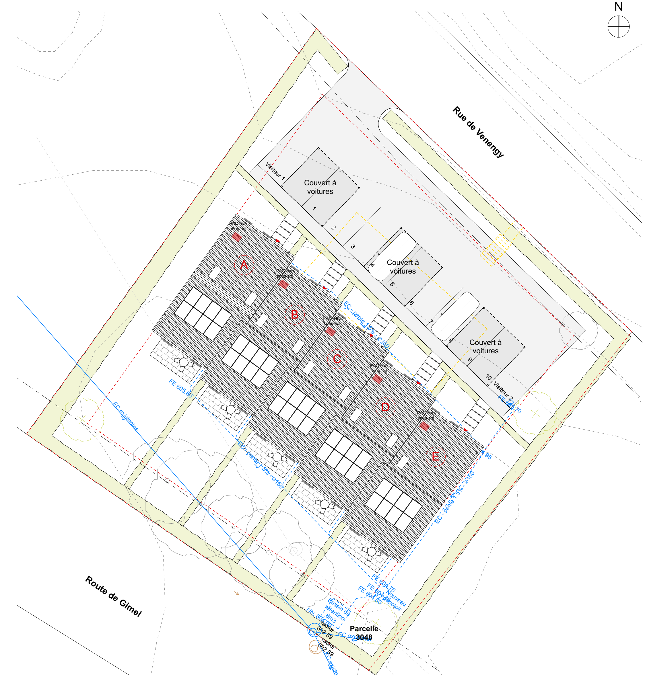
PLAN DE SITUATION
