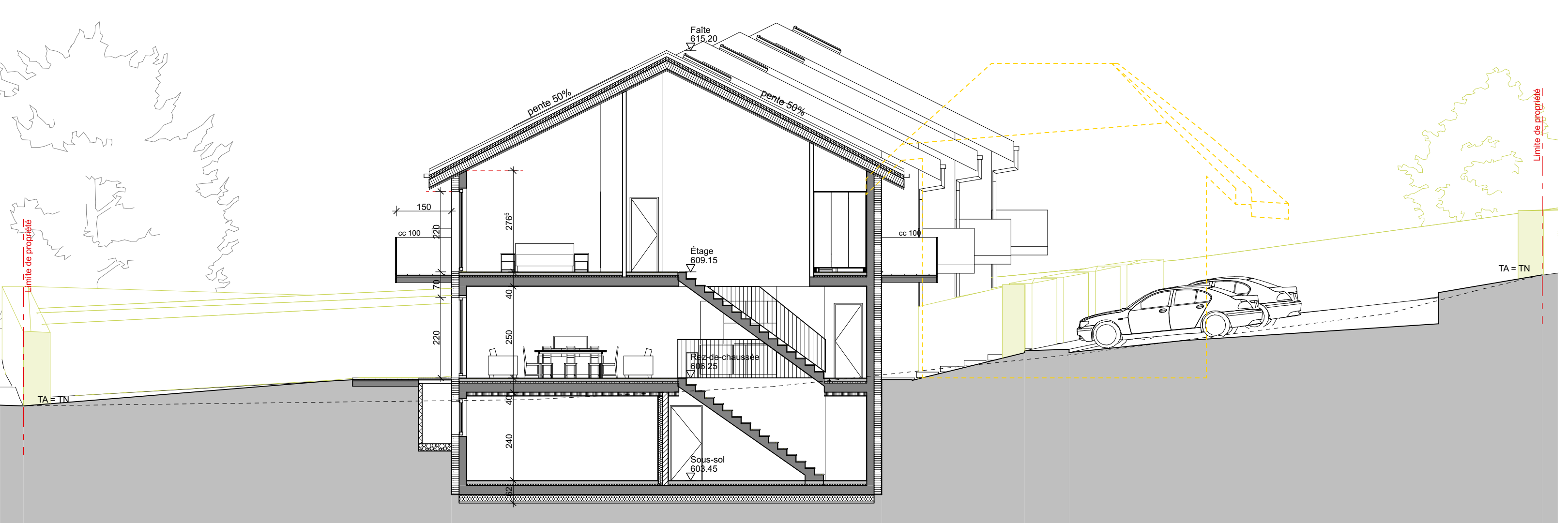
COUPE TRANSVERSALE TYPE
